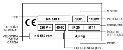
Placa de características
