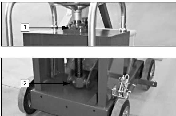
5.4.1-2 Schmierpunkte der Höhenverstellungsschraube
