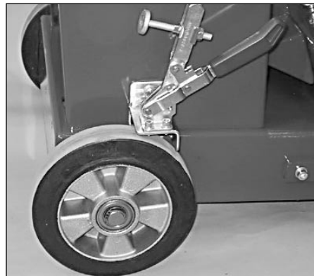
Abb. 7.3. Feststellbremse gelöst
