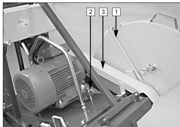
5.2.1. Wasserrohr für Kühlung der Schneidklinge
