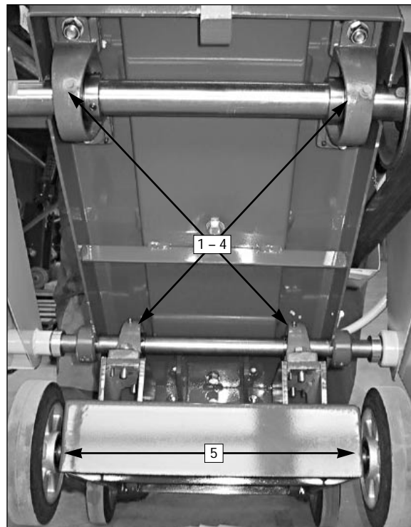
5.1.1-4 Schmierpunkte der Lagerböcke
