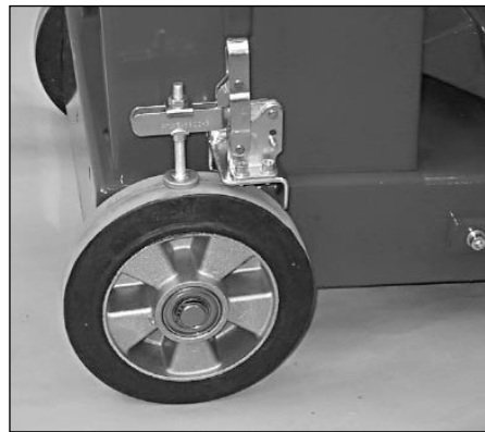
Abb. 7.2. Feststellbremse eingeschaltet
