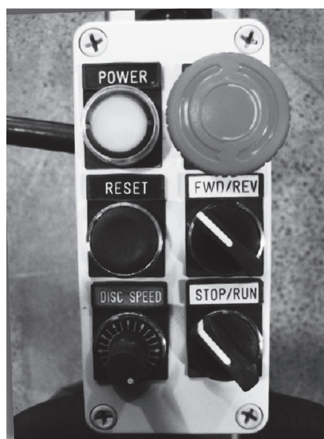
Manöverpanel
