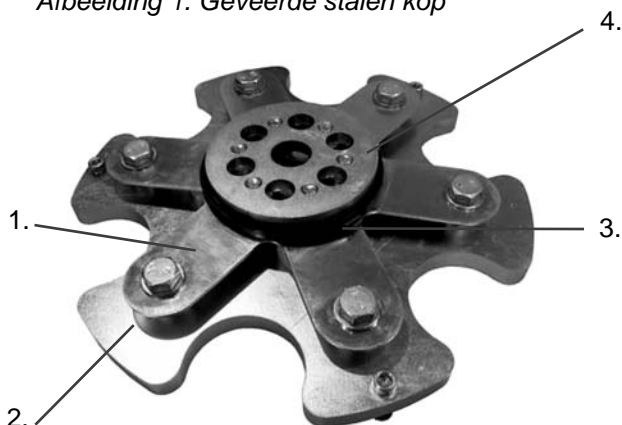
Afbeelding 1. Geveerde stalen kop
