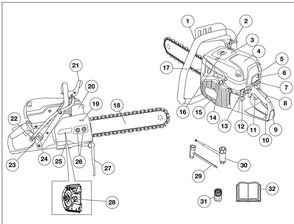
Componentes de la máquina - K970 III Chain
